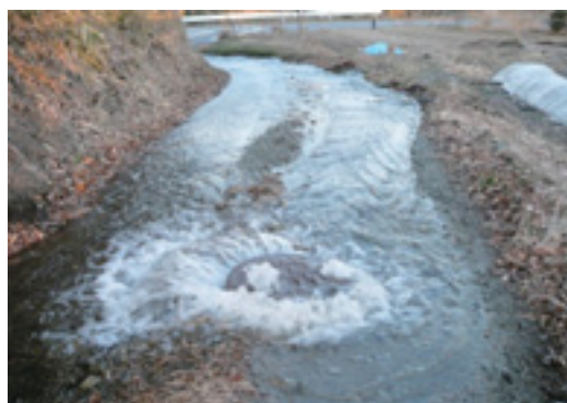
空気弁からの漏水
